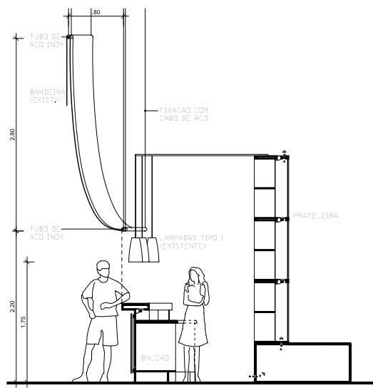
Teilschnitt Empfangsbereich
